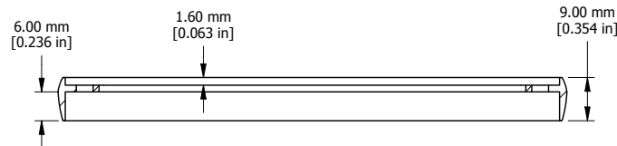
OPEN BEZEL
