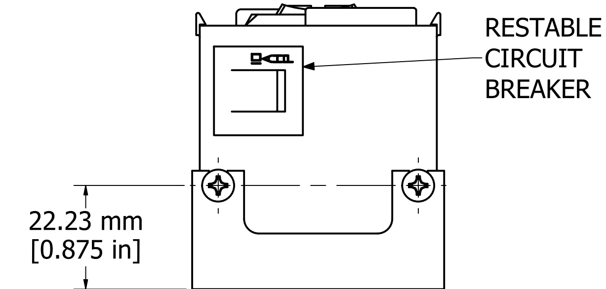
VIEW A-A
