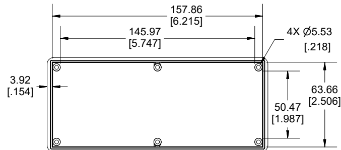
INSIDE LID
