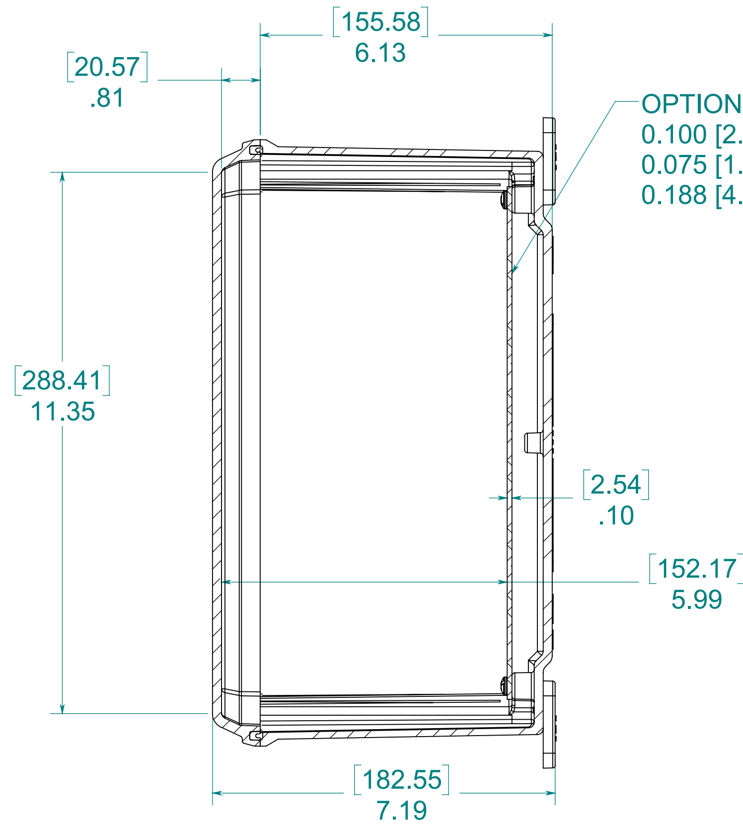
SECTION A-A
