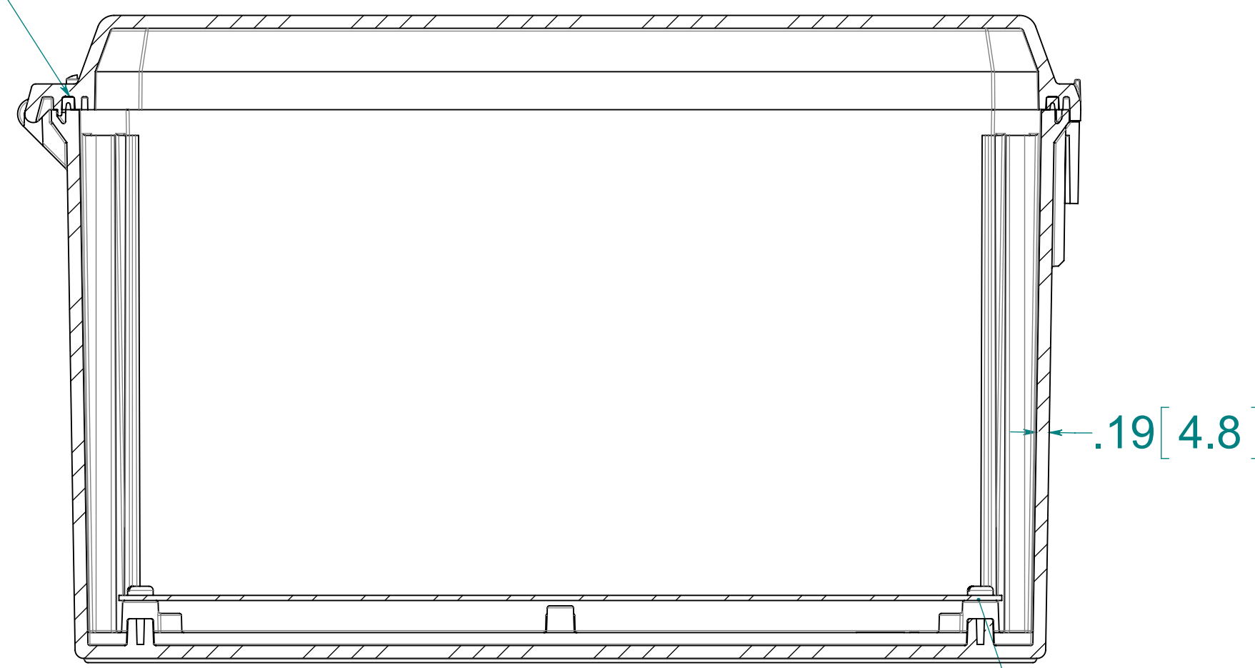
SECTION D-D
