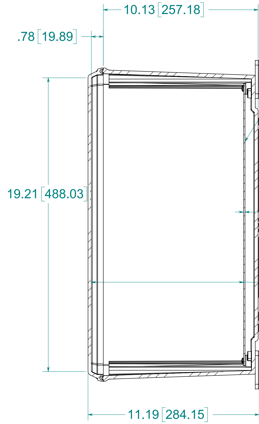
SECTION A-A
