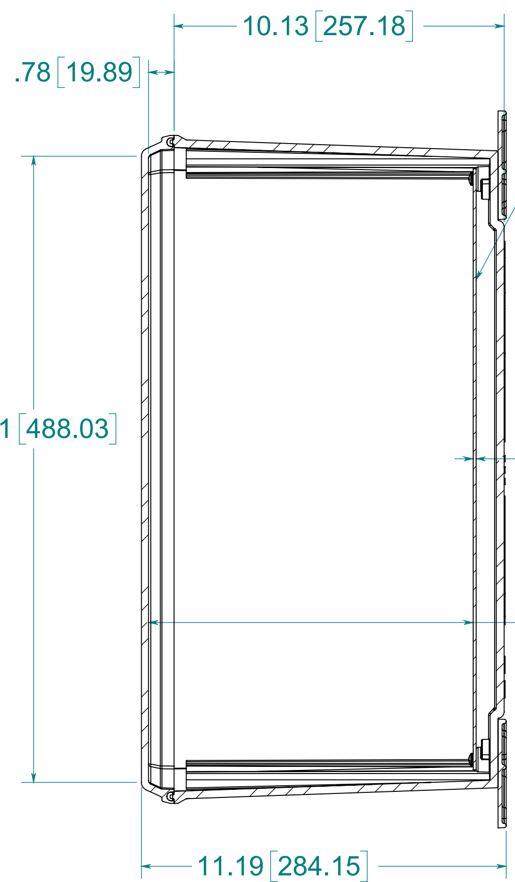
SECTION A-A
