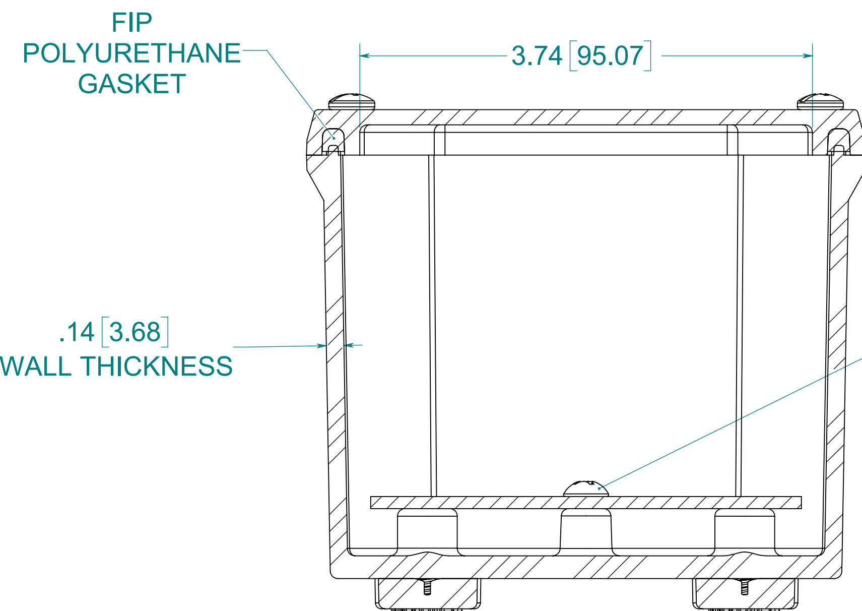
SECTION A-A
