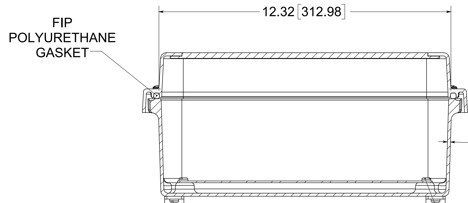
SECTION A-A
