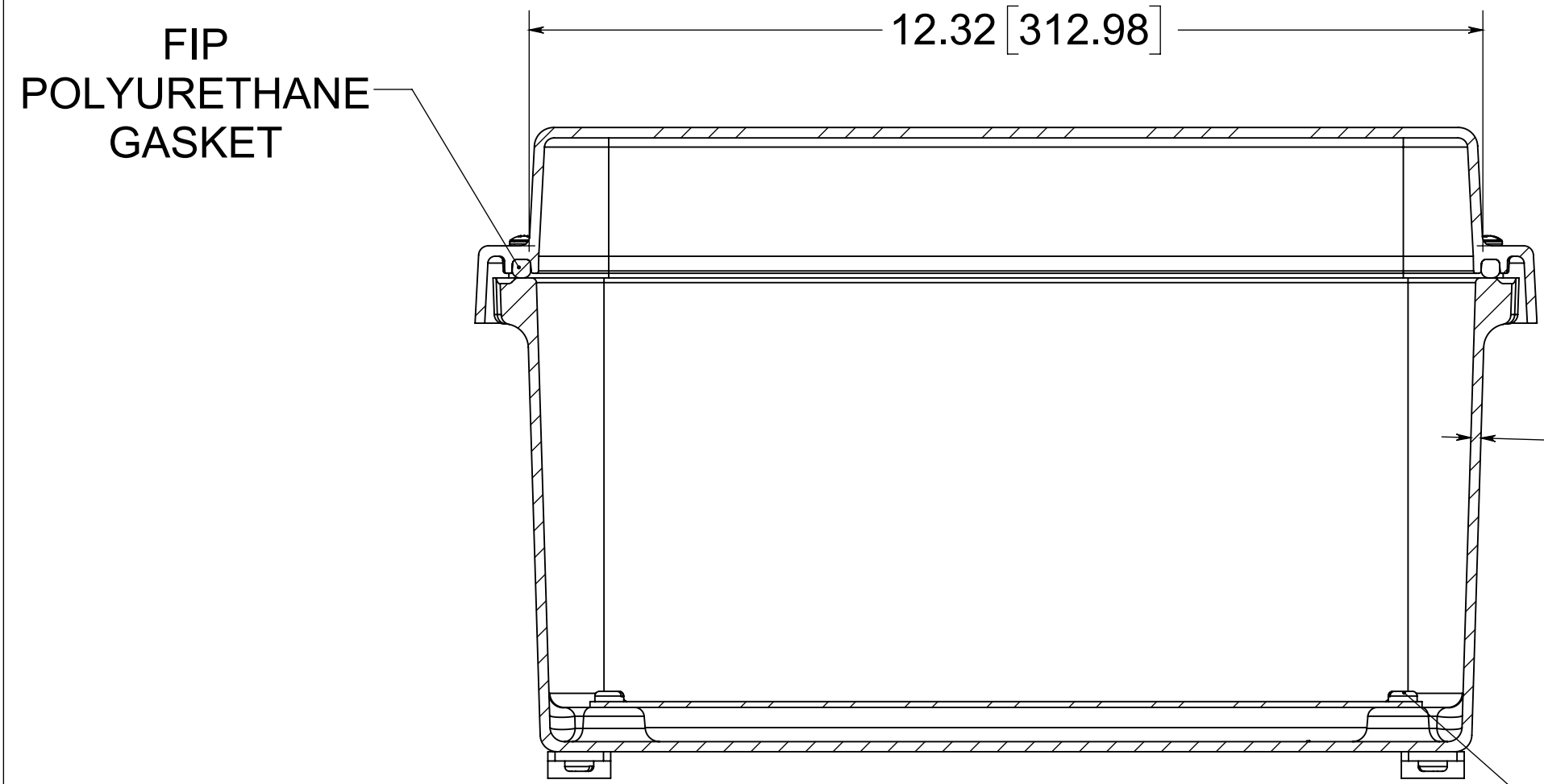
SECTION A-A
