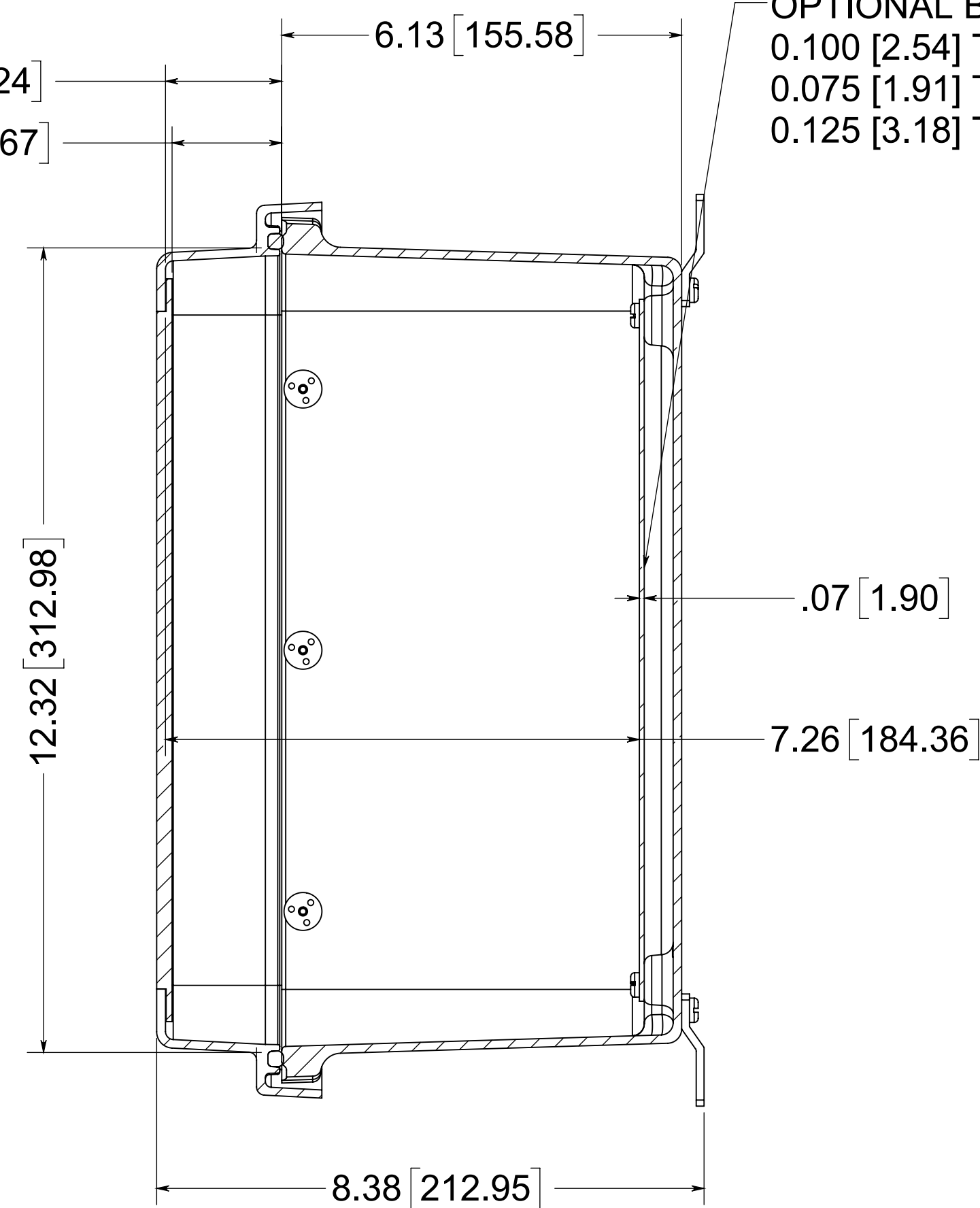
SECTION A-A
