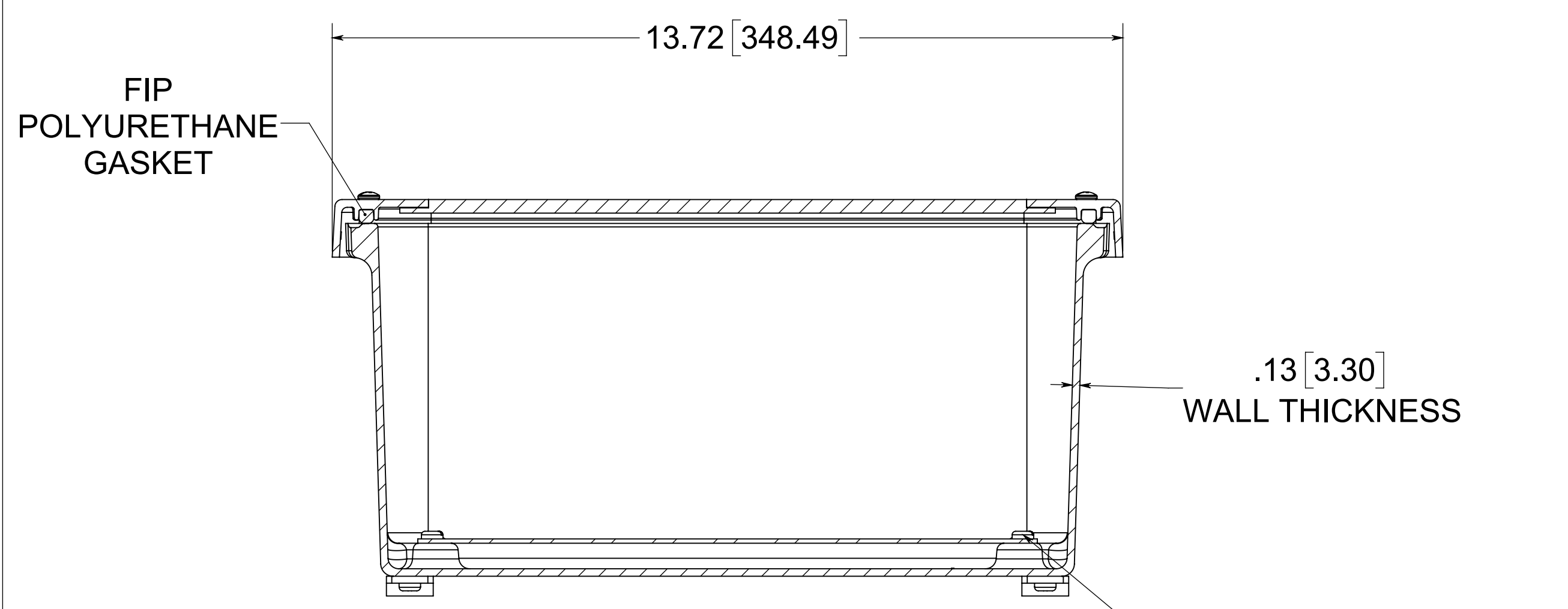
SECTION A-A
