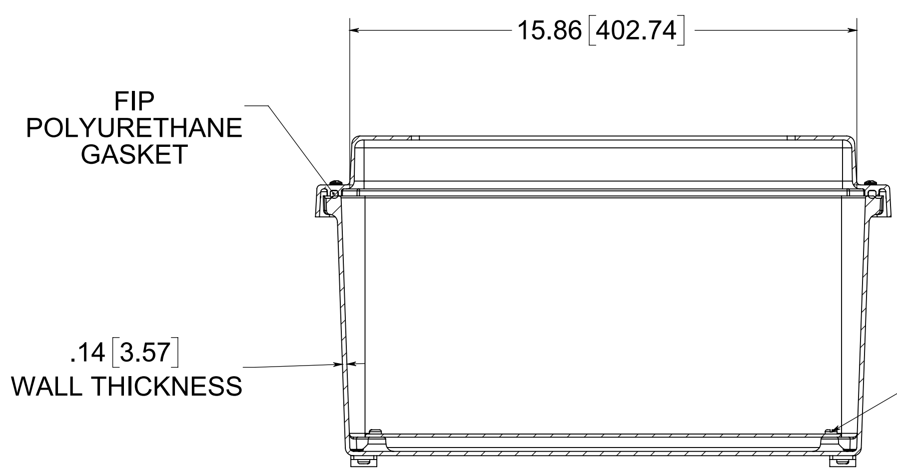
SECTION A-A
