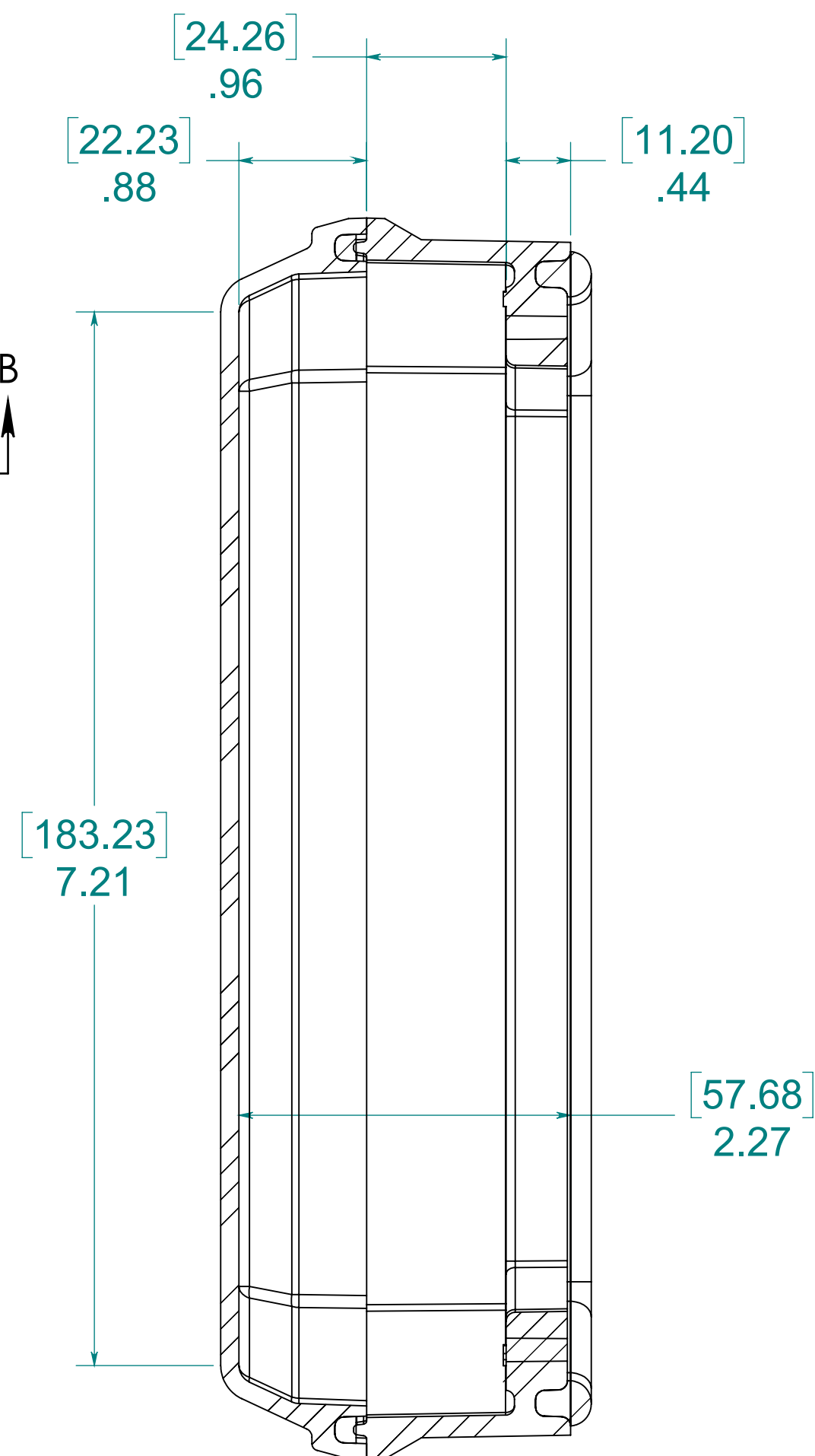
SECTION A-A
